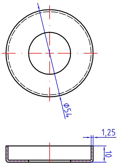
Innenteil mit Olive (inside part with olive knob)
