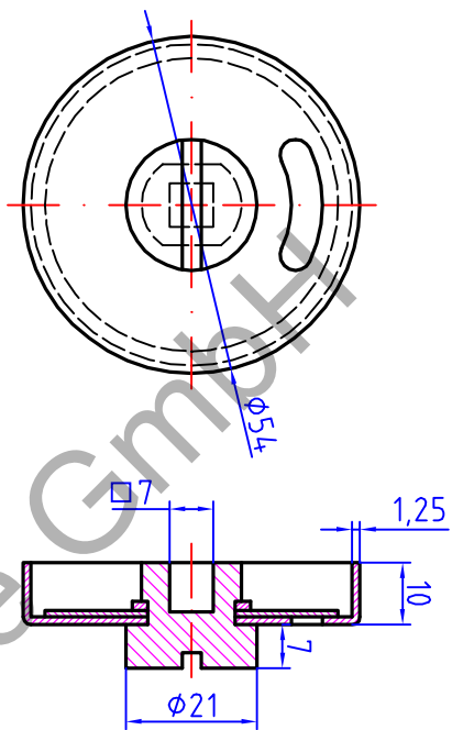
Außenteil mit rot/grün-scheibe (outside part with red/green sign)
